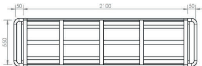
Tampak Atas
